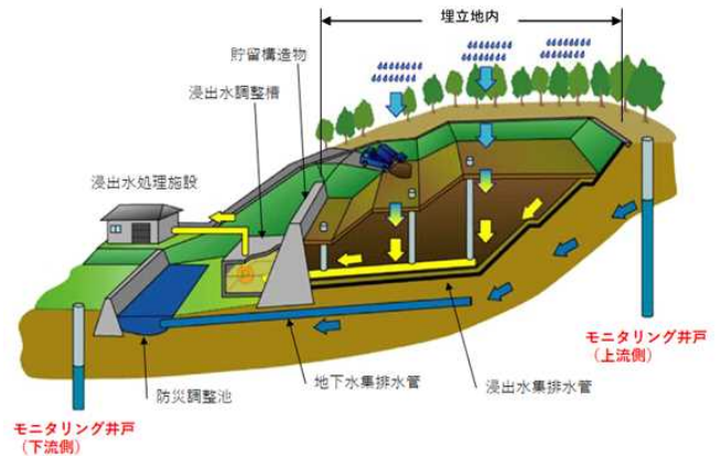
図 1 最終処分場（オープン型）のイメージ図
