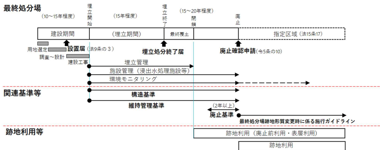
図 1-4 最終処分場の整備から閉鎖・廃止までの流れ
